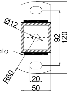
DETTAGLIO PIASTRA MONTANTE
